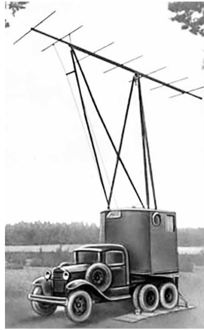
Одна из первых передвижных станций РУС-2
